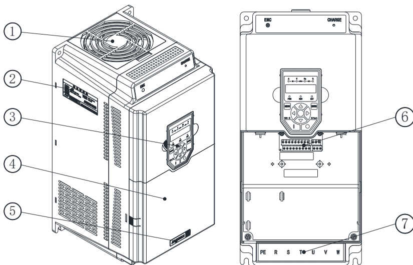
Hope150PM30T4D~37T4D-产品部件示意图
