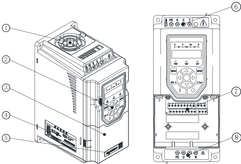
Hope150PM5.5T4U~7.5T4U、Hope150PM4S2U 产品部件示意图
