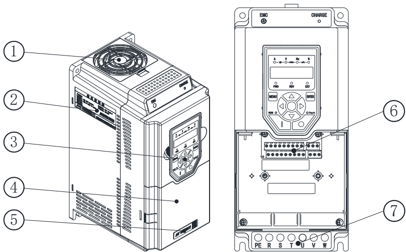
Hope150PM11T4D~15T4D-产品部件示意图
