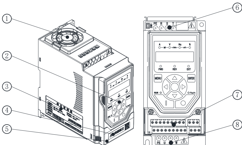
Hope150PM0.75T4U~4T4U、0.75S2U~2.2S2U 产品部件示意图
