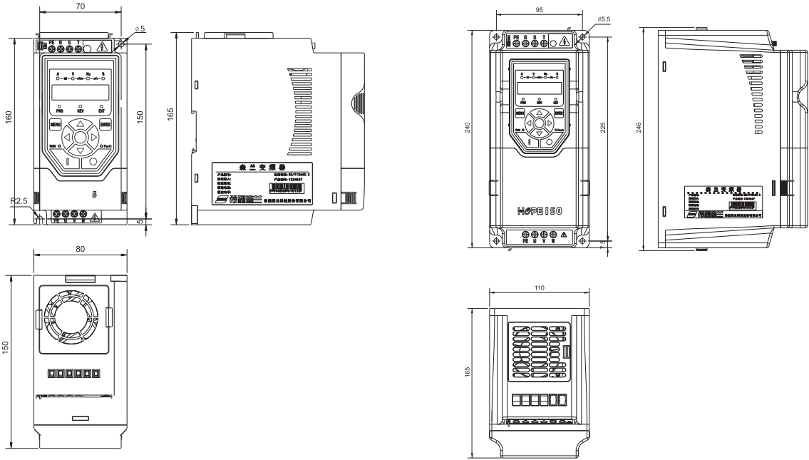
Hope150G0.75T4U~4T4U、0.75S2U~2.2S2U上进下出线机型外形图和尺寸如下：
